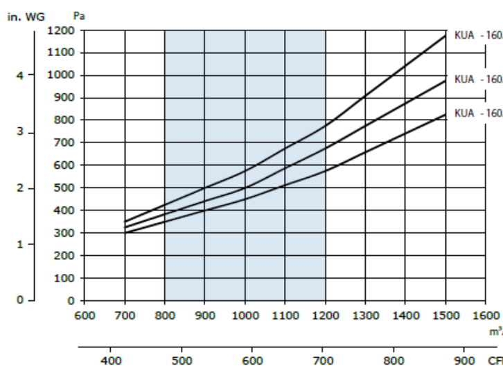
Grafico delle perdite di carico
