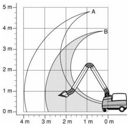
Raggio d'azione Ultraflex 3 (B) – Ultraflex 4 (A) su filtro carrellato
