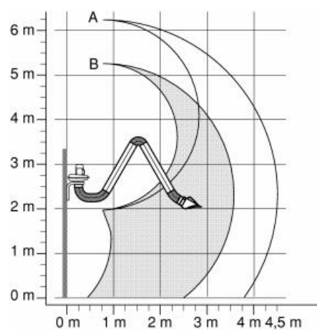
Raggio d'azione Ultraflex 3 (B) – Ultraflex 4 (A) a parete
